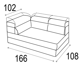
102 166 108 terminale ad angolo senza pouf dx-sx right-left terminal corner without pouf
